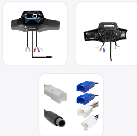
Pantalla, vista trasera y conectores
