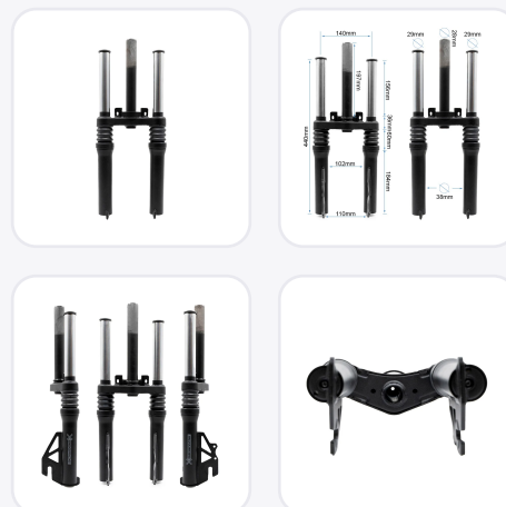
Vues de l'amortisseur et dimensions
