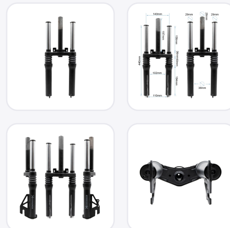
Viste dell'ammortizzatore e dimensioni
